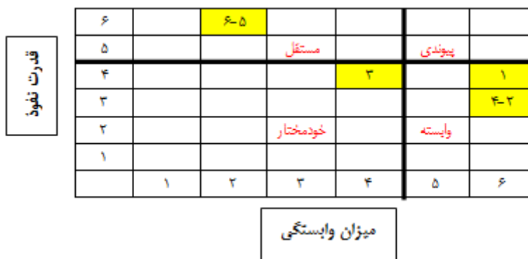
نمودار ۲- ماتریس قدرت نفوذ- وابستگی یا تحلیل MICMAC Figure 2. MICMAC dependency- penetration power matrix or analysis
