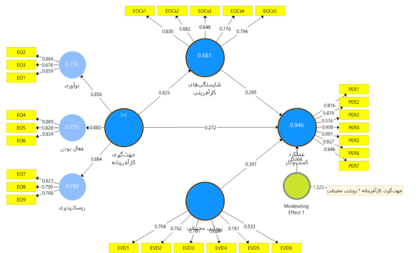
شکل ۲- ضرایب مسیر مدل Figure 2. Model path coefficients
