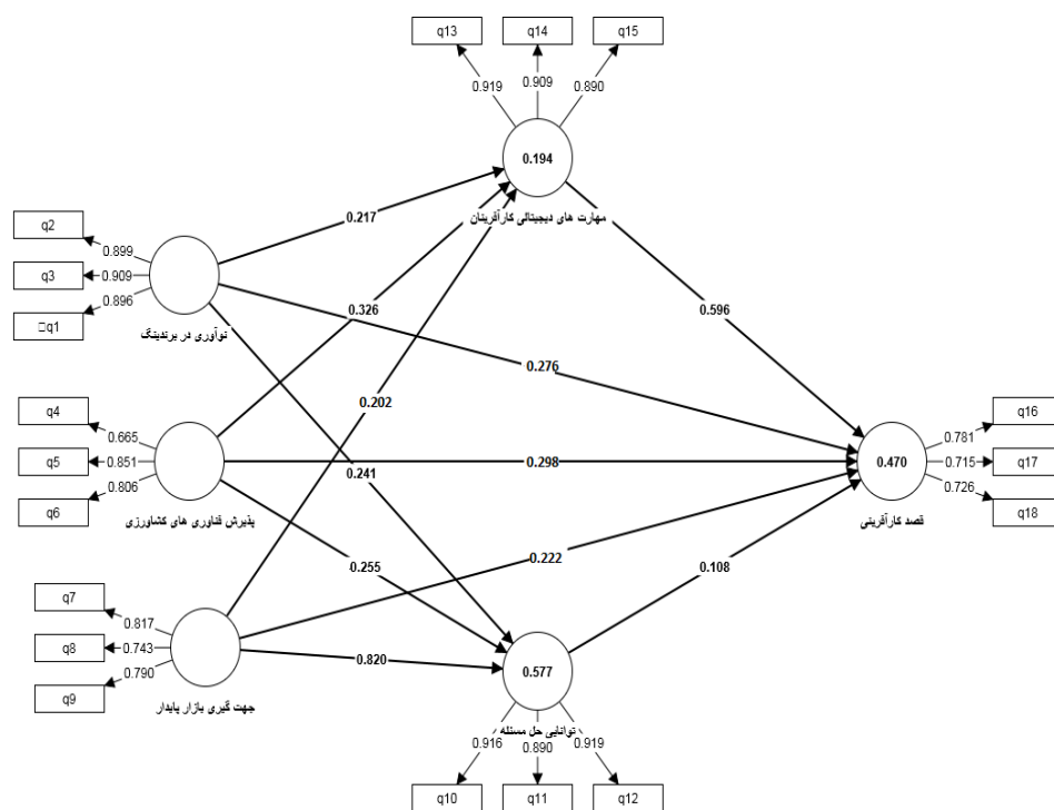
شکل ۳- مدل سازی معادلات ساختاری در حالت استاندارد Figure 3. Structural equation modeling in the standard mode
