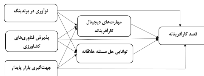
شکل ۱- مدل مفهومی پژوهش Figure 1. Conceptual research model
