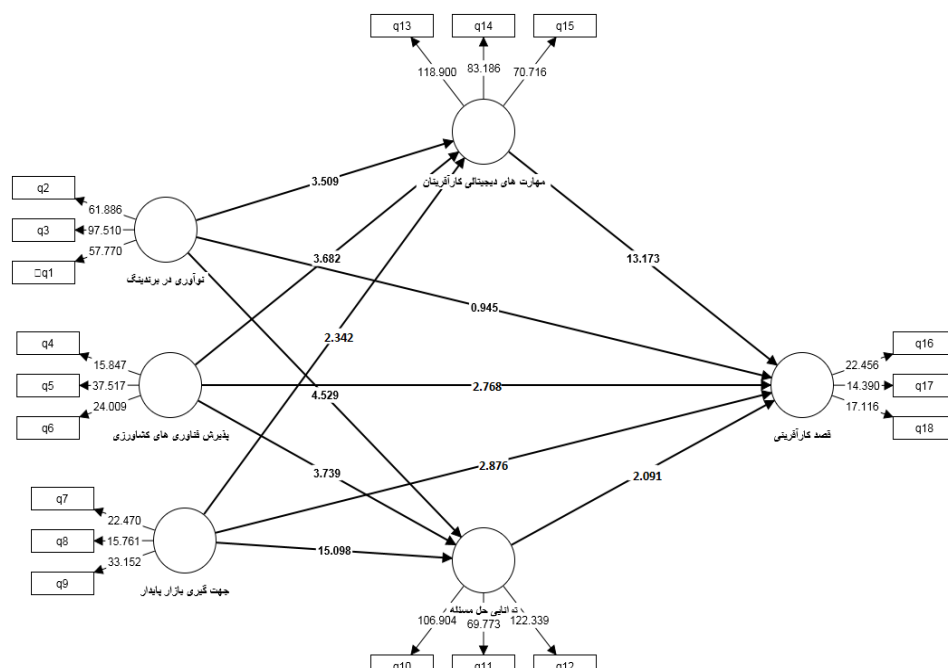
شکل ۲- مدل سازی معادلات ساختاری در حالت معناداری Figure 2. Structural equation modeling in the significant mode
